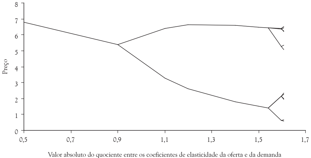
Figura 4. Bifurcações obtidas por meio de um modelo linear de oferta e demanda com antecipações adaptativas de preços. Fonte: simulações elaboradas pelo autor a partir do modelo descrito em Silva Neto (2004).
