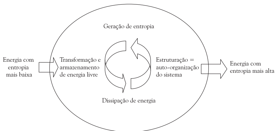
Figura 1. Esquema geral de um sistema dissipativo que se mantém longe do equilíbrio. Fonte: elaborado pelo autor.
